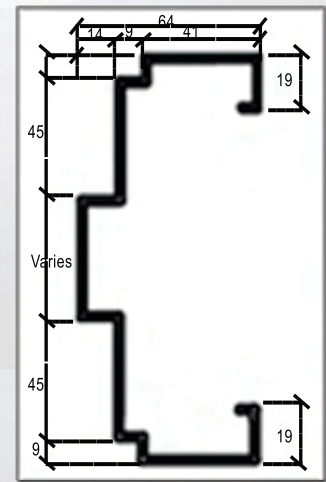
Double Rabbet Frame Ind'l Des. Reg. 3-2004-000520
