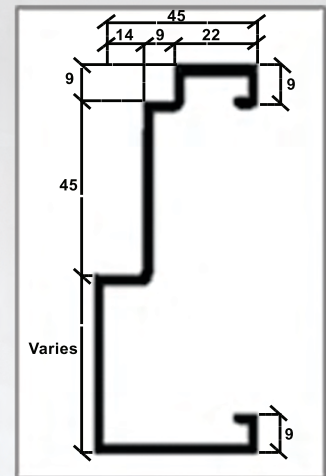
Single Rabbet Frame Ind'l Des. Reg. 3-2004-000519
